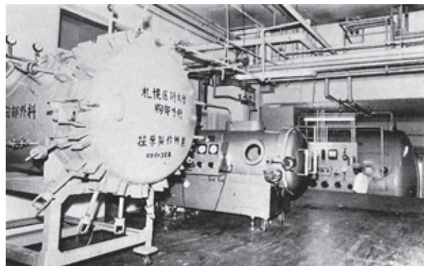
札幌医科大学の高気圧治療装置
